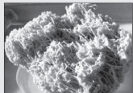
კალციტი (ტრაპერტინი), ნახჭევანი
