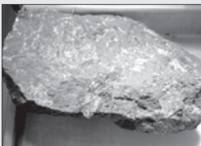
ლაზრაფორიტი, მდინარე ლიახვის ხეობა
